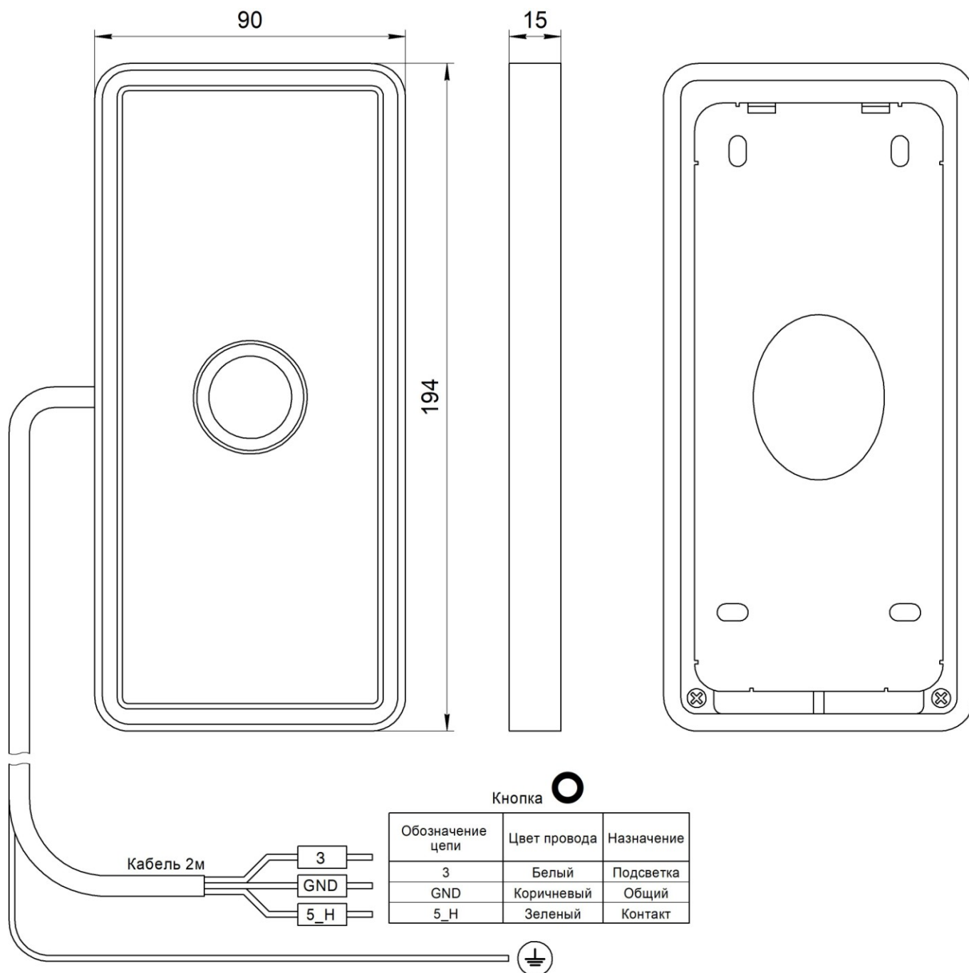
Рис.1 Внешний вид и габаритные размеры Вызывного поста ОБСИДИАН НШЕК.468381.215
